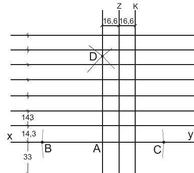
Obr. 1 - Rozvržení krytiny
