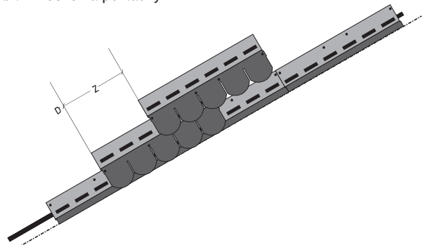
Obr. 4 - Schéma pokládky
